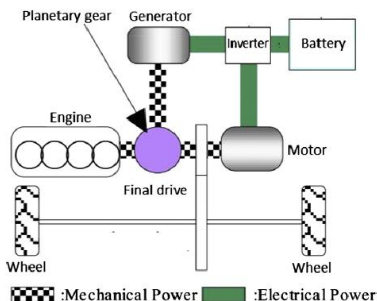
Hình 1. Mô hình xe lai phân chia công suất [12]
