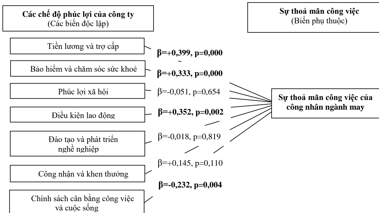
Hình 2. Mô hình hồi quy tuyến tính đa biến.
