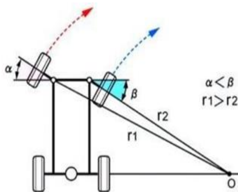
Hình 6. Ô tô khi quay vòng
