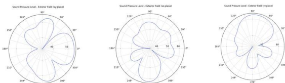
Hình 20. Đồ thị áp suất âm thanh biểu thị theo phương XY, XZ, YZ ở tốc độ quay 5000v/p
