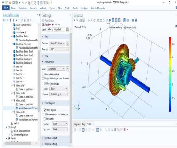
Hình 7. Phân tích độ rung của vi sai
