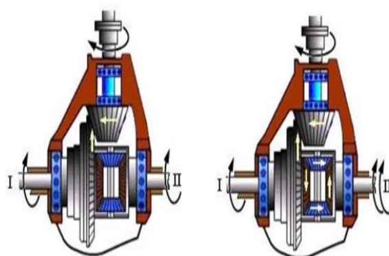
Lực cản trục I bằng trục II (a) Khi chạy thẳng Lực cản trục I lớn hơn trục II (b) Khi quay vòng
