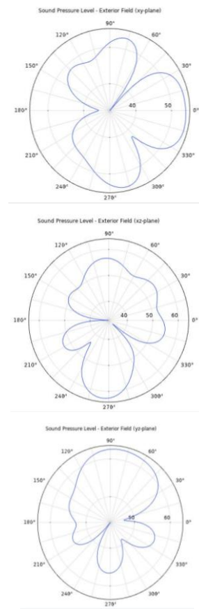
Hình 10. Đồ thị biểu thị áp suất âm thanh theo phương XY, XZ, YZ
